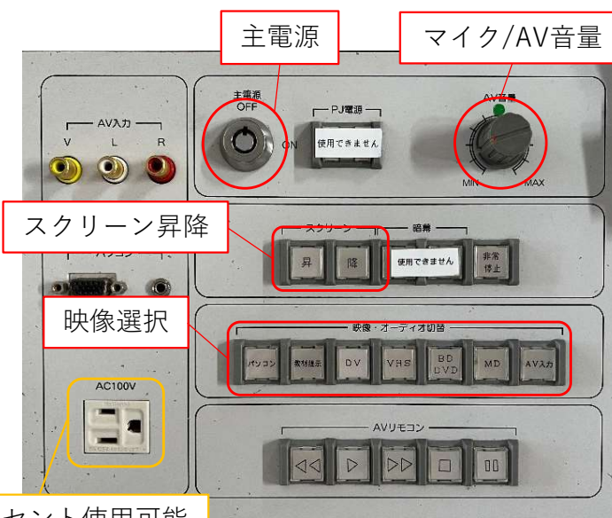
操作パネル
